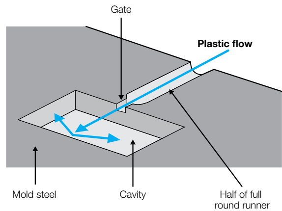
Figure 9.23 Edge gate
